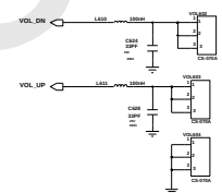
Volmue Key
